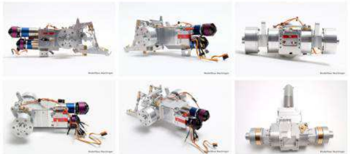
Abbildung 125: 2-Gang Getriebe, verschiedene Ausbaustufen in 1:16
