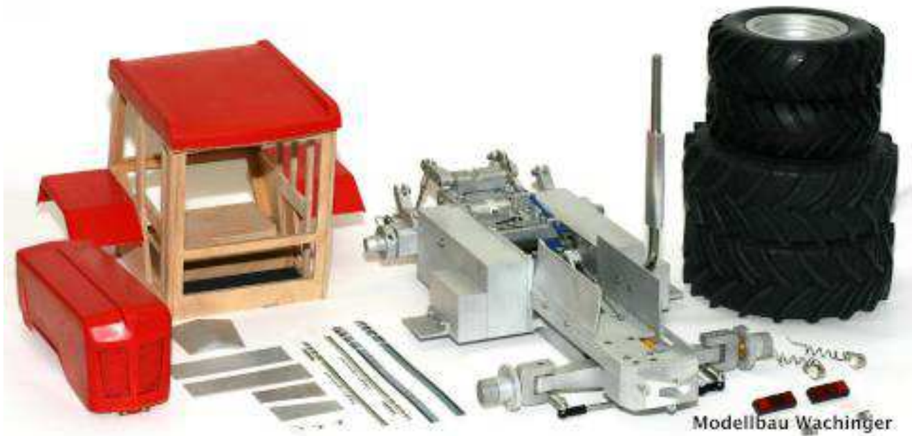
Abbildung 16: Teile des Bausatzes
