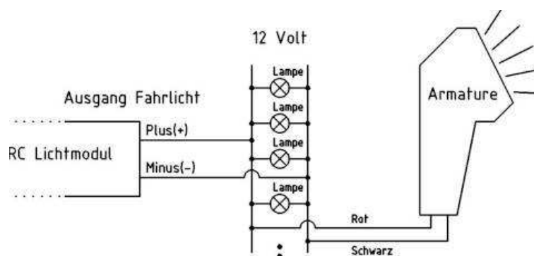
Abbildung 136: Vorschlag zur Verdrahtung
