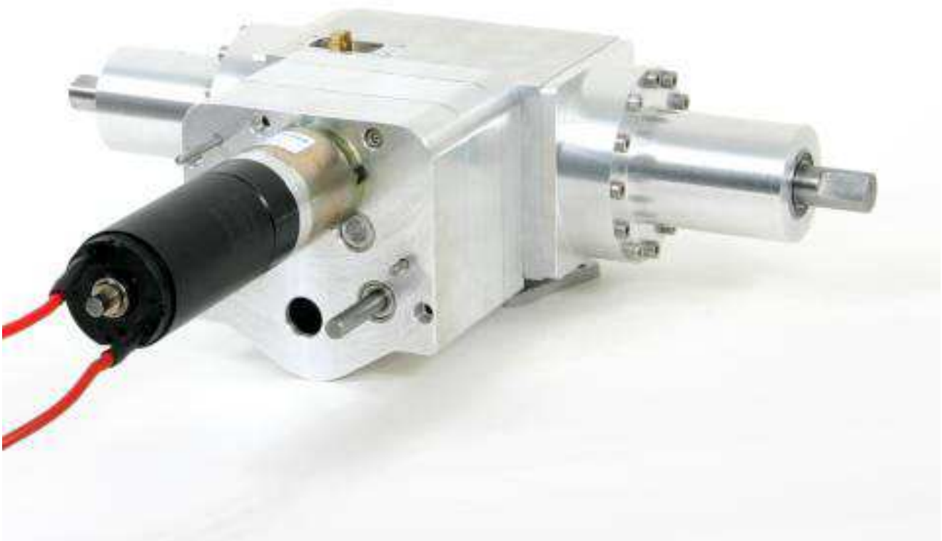
Abbildung 44: 2-Gang Getriebe
