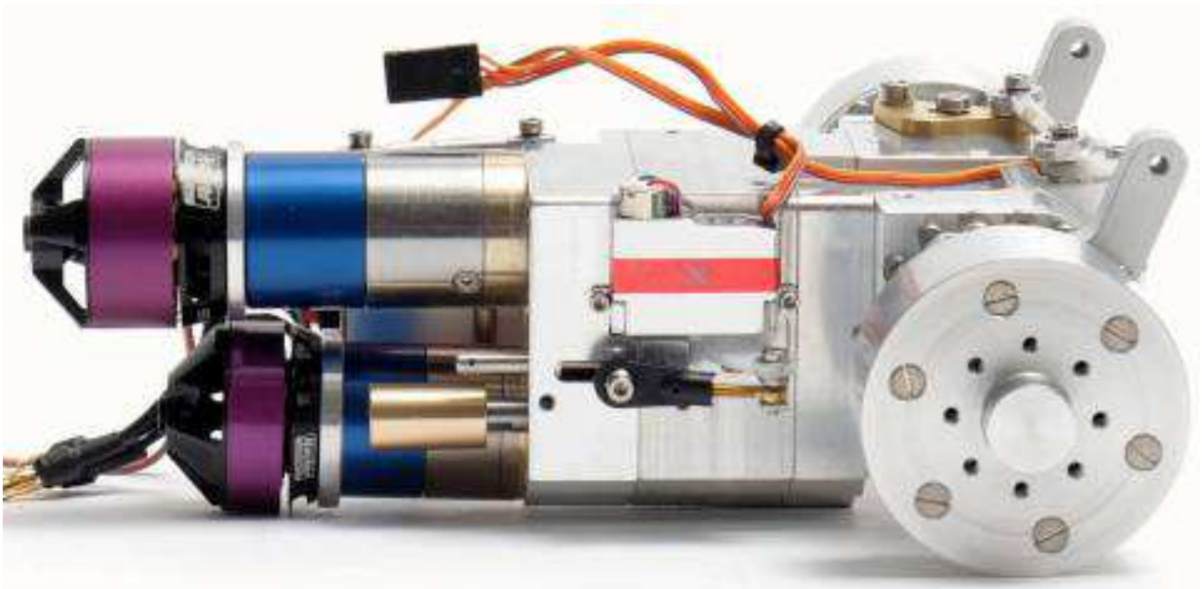
Abbildung 116: 2-Gang Getriebe, verschiedene Ausbaustufen in 1:14.5
