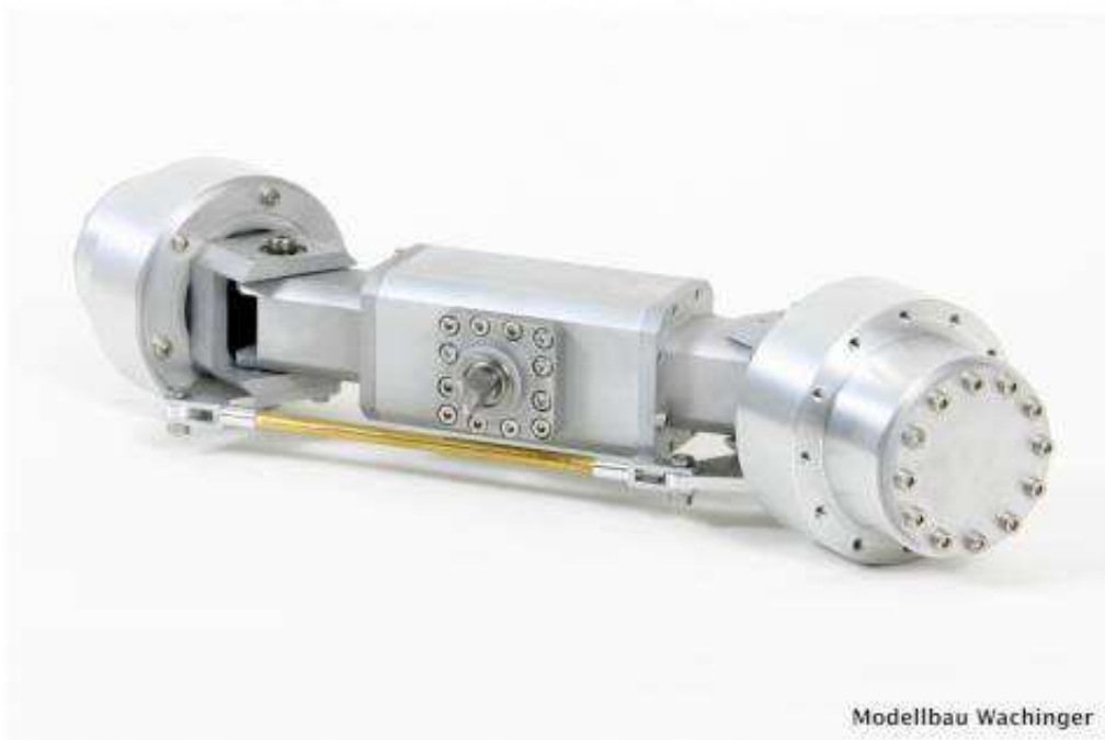
Abbildung 41: Vorderachse Planetengetriebe
