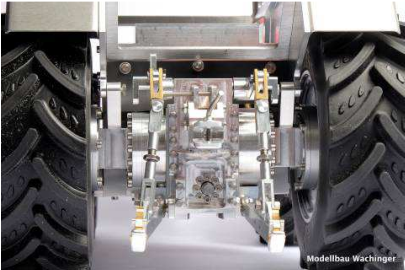
Abbildung 128: Dreipunkt Aufhängung 1:16
