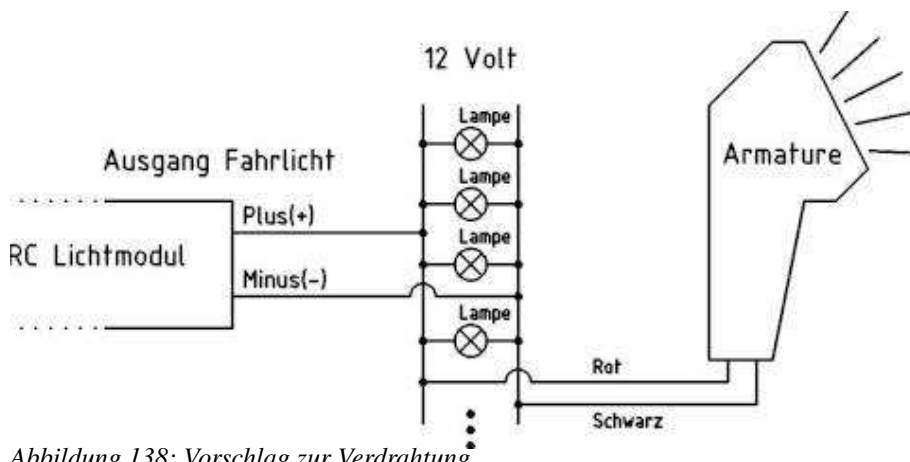
Abbildung 138: Vorschlag zur Verdrahtung
