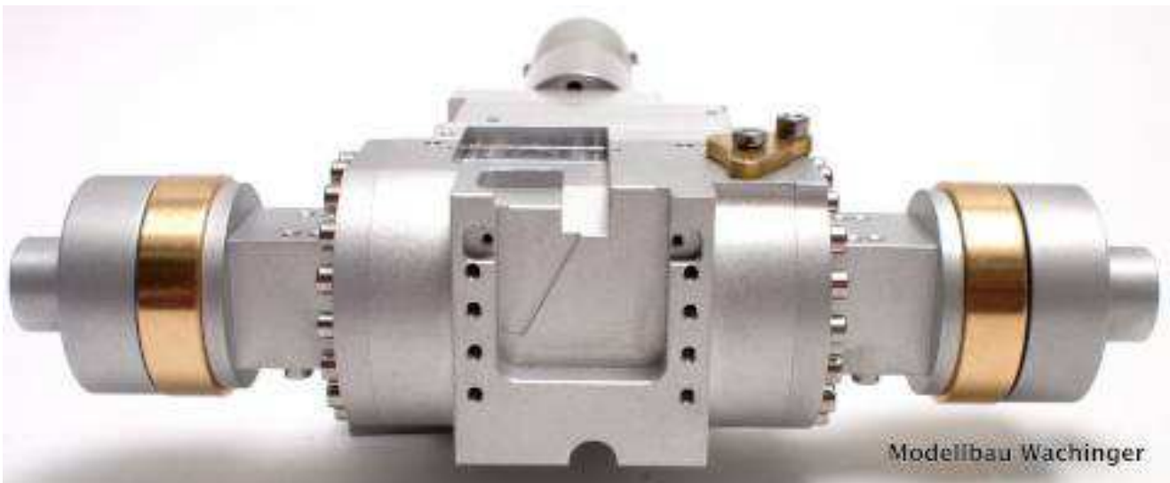
Abbildung 126: 2-Gang Getriebe, verschiedene Ausbaustufen in 1:16
