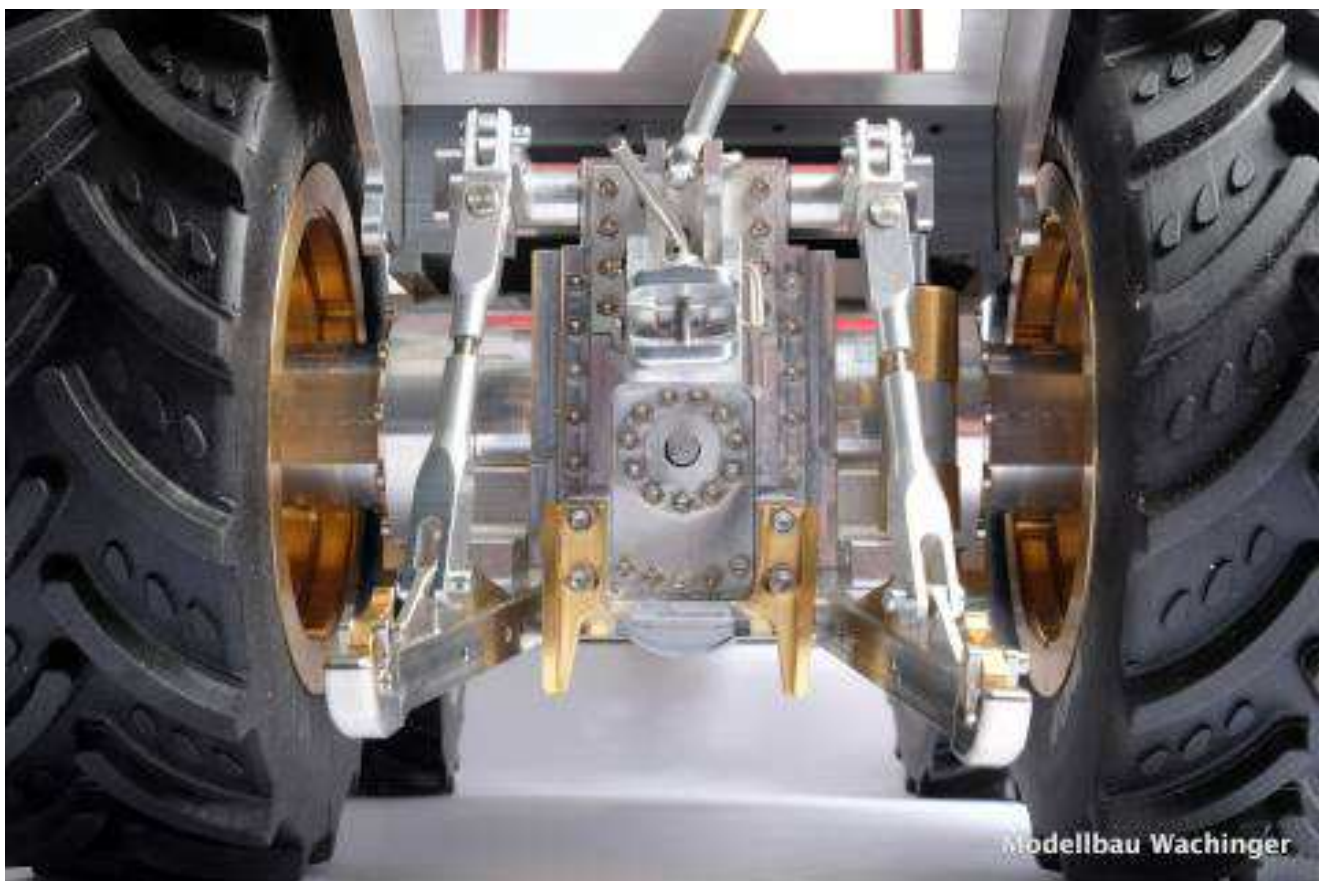
Abbildung 18: Details des Chassis
