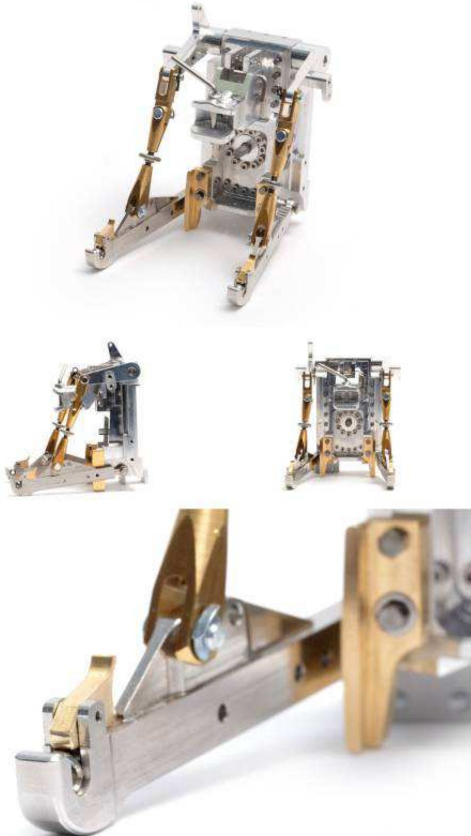
Abbildung 49: Dreipunkt Aufhängung
