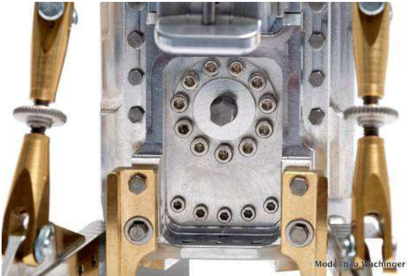
Abbildung 50: Dreipunkt Aufhängung
