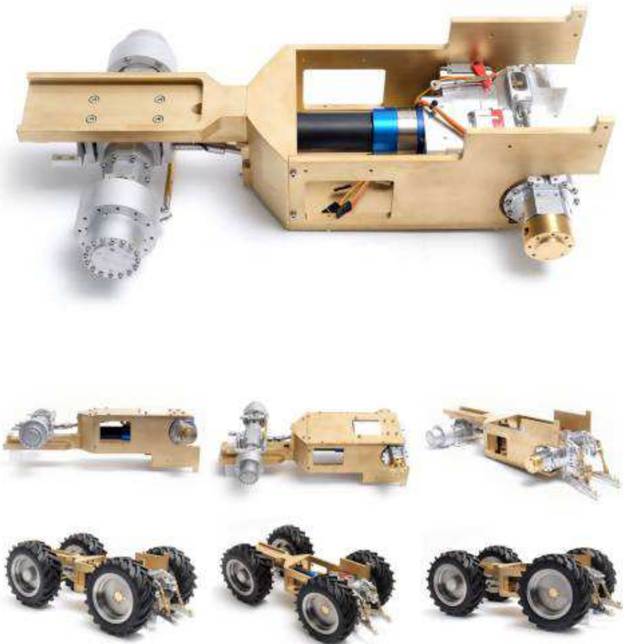
Abbildung 27: Ein Messing Chassis!
