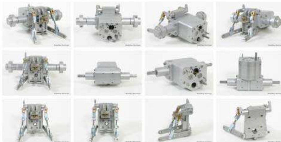
Abbildung 105: Getriebe
