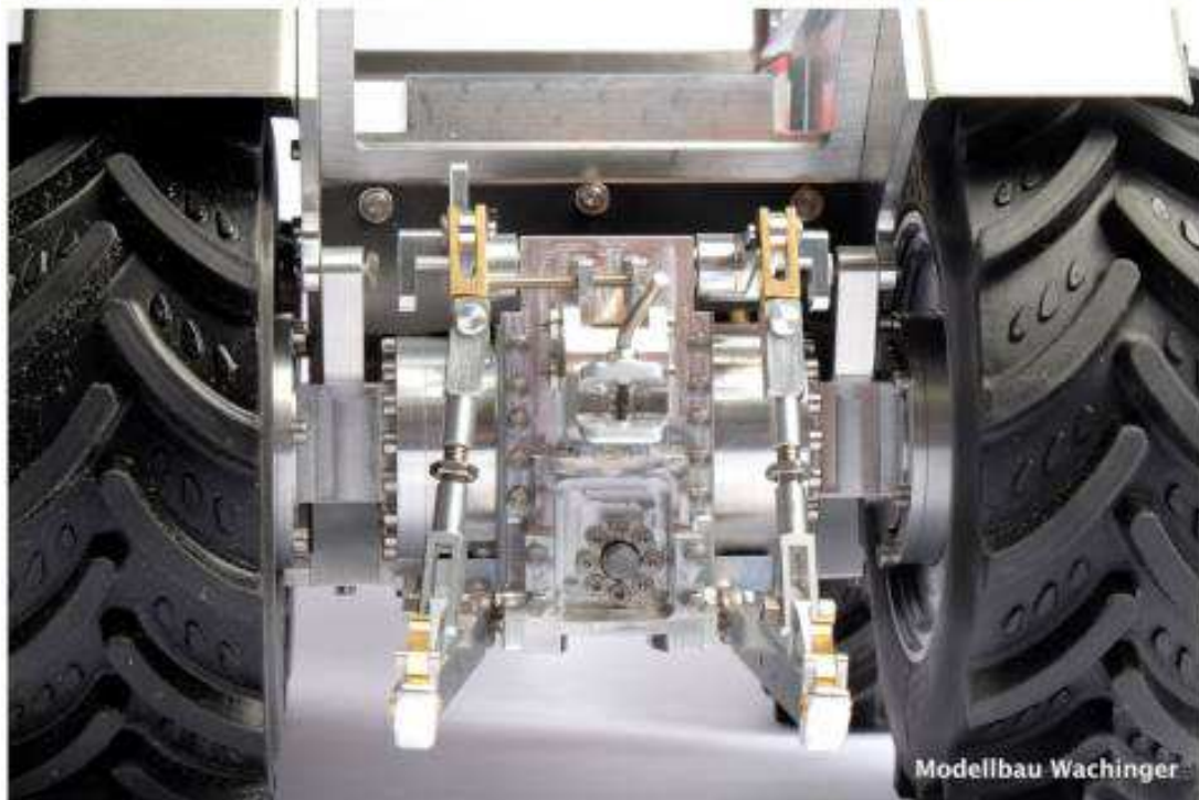
Abbildung 109: Bausatz 2000 TVL, neues Modell
