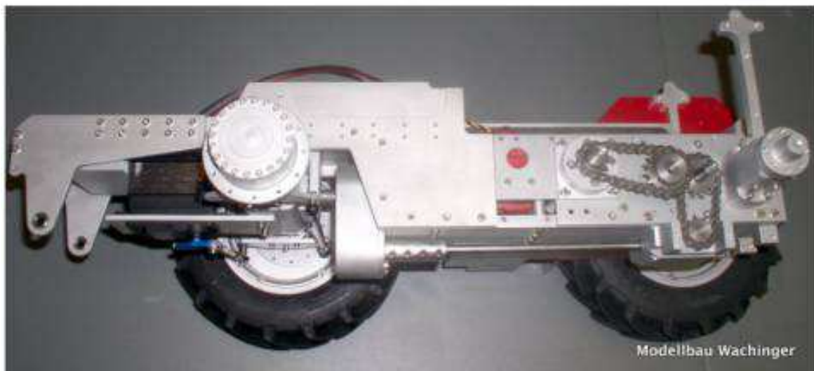
Abbildung 38: Vorderachse Allrad
