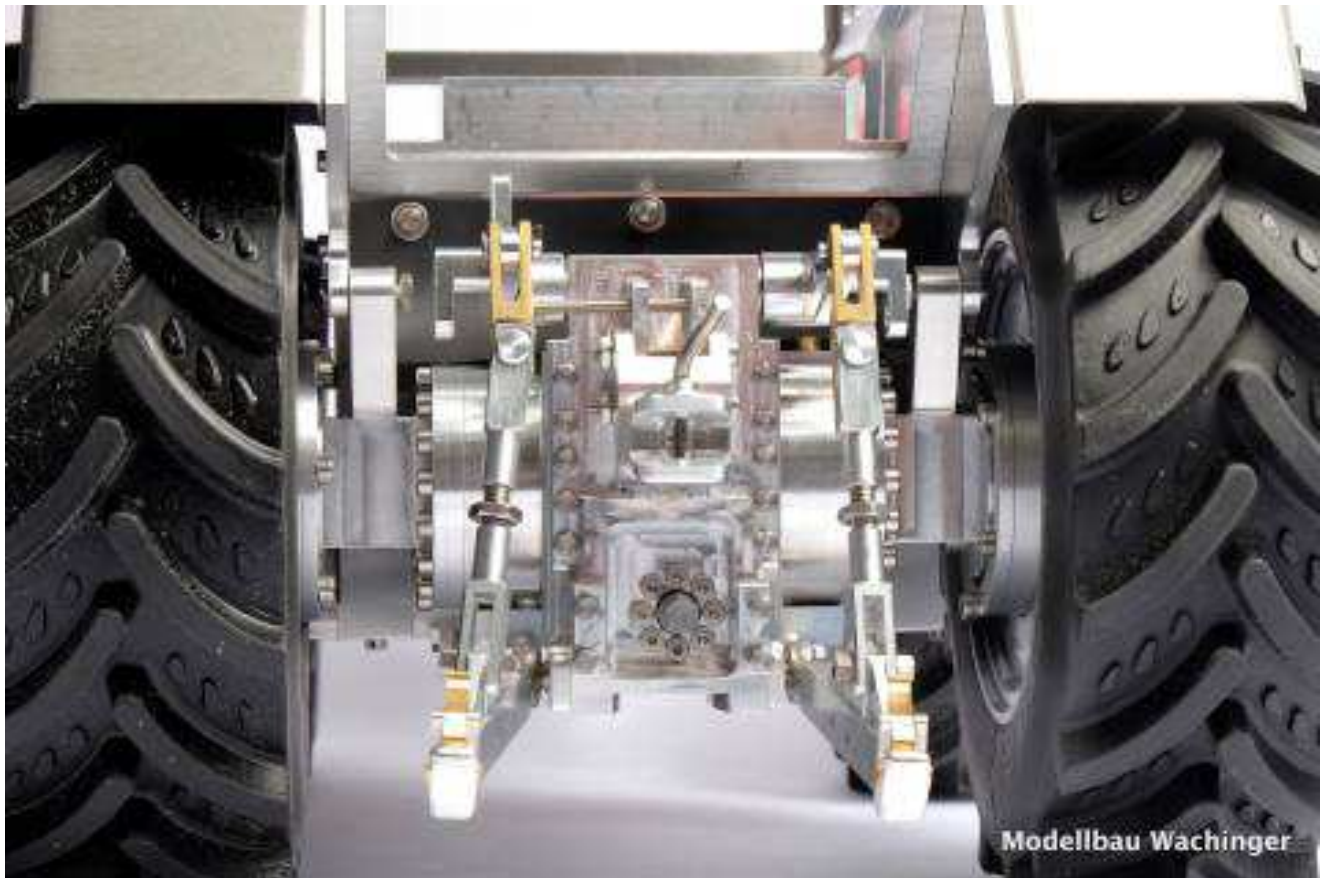
Abbildung 118: Dreipunkt Aufhängung Beispiel
